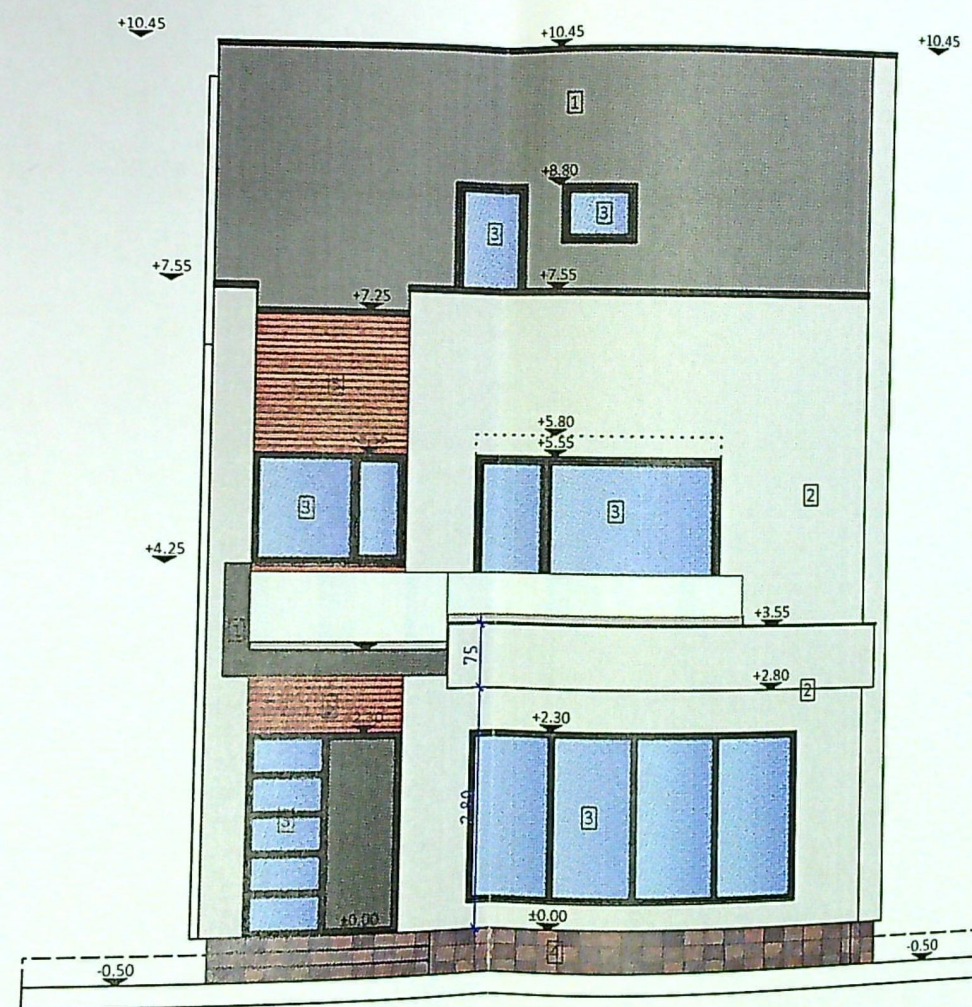
FATADA NORD-VEST
